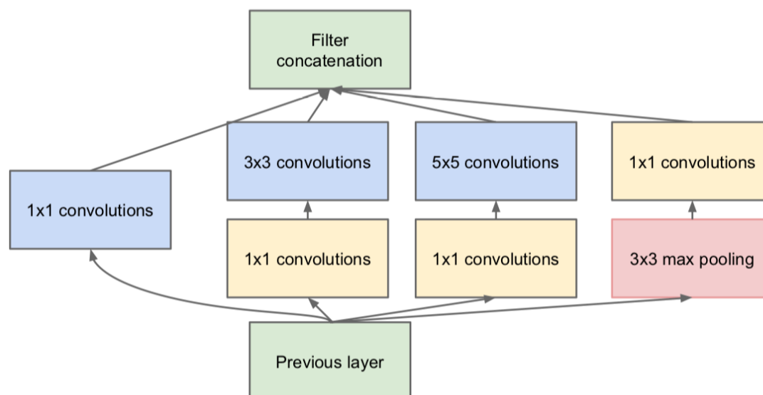
Fig. 5: Inception Module
