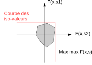
FIG. 2: Polyèdre des valeurs possibles des fonctions objectives ( |\mathbf{S}|=2 ) cas 2
