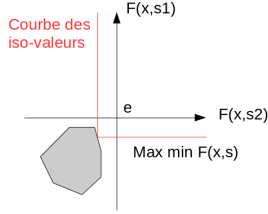
FIG. 1: Polyèdre des valeurs possibles des fonctions objectives ( |\mathbf{S}|=2 ) cas 1
