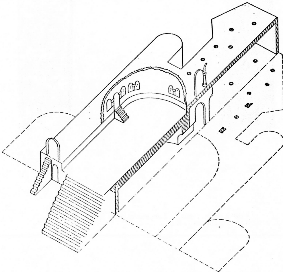
Flavigny, église abbatiale Saint-Pierre, coupes longitudinale et transversale et vue diagrammatique du chevet, par C. MALONE (Harvard-Berkeley).
