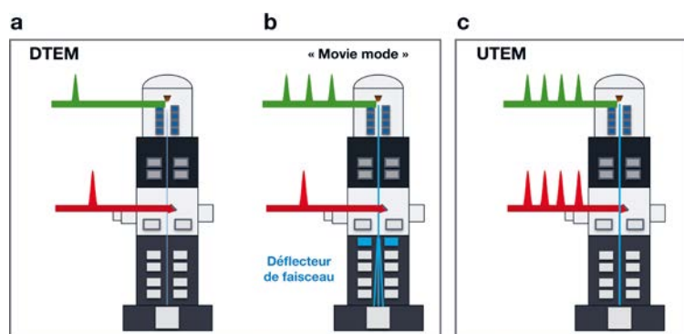
Figure 2. Les deux types de microscopes électroniques résolus en temps : les DTEM (Dynamic Transmission Electron Microscope) et les UTEM (Ultrafast Transmission Electron Microscope).
