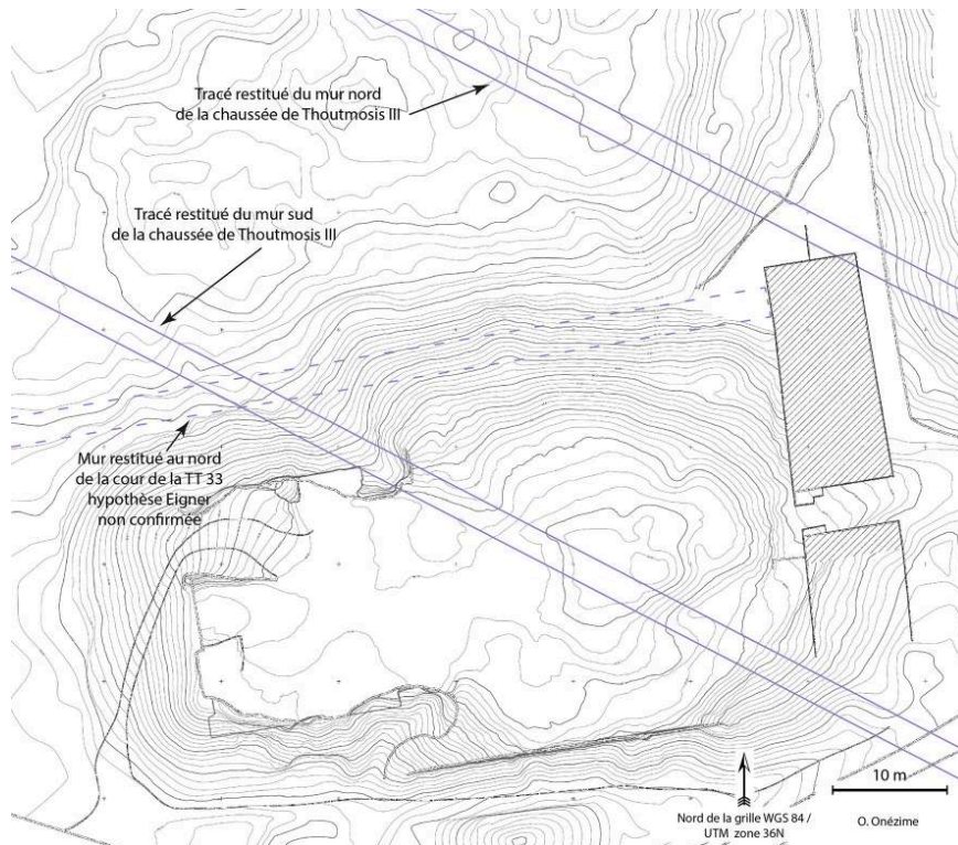
Fig. 1. Intersection de la chaussée de Thoutmosis III et du pylône de la TT 33 (plan O. Onézime, Fr. Colin, 2018).
