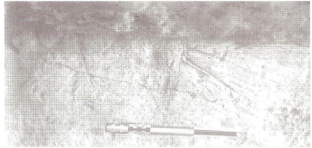
Fig. 18 – Empreintes de roseaux pris dans le mortier de djousse , sur le socle de la courtine.
