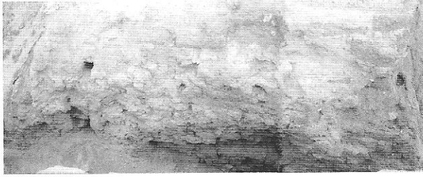
Fig. 29 - Coupe sur le sommet du rempart ; au centre, le mur B4.
