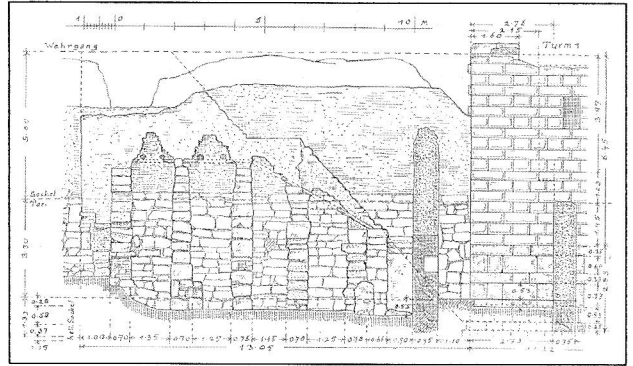
Fig. 10 – Dessin de A. von Gerkan : le rempart contre la tour 1. En haut à droite, sondage opéré par von Gerkan. Prel. Rep. VII-VIII , p.57, fig.26.
