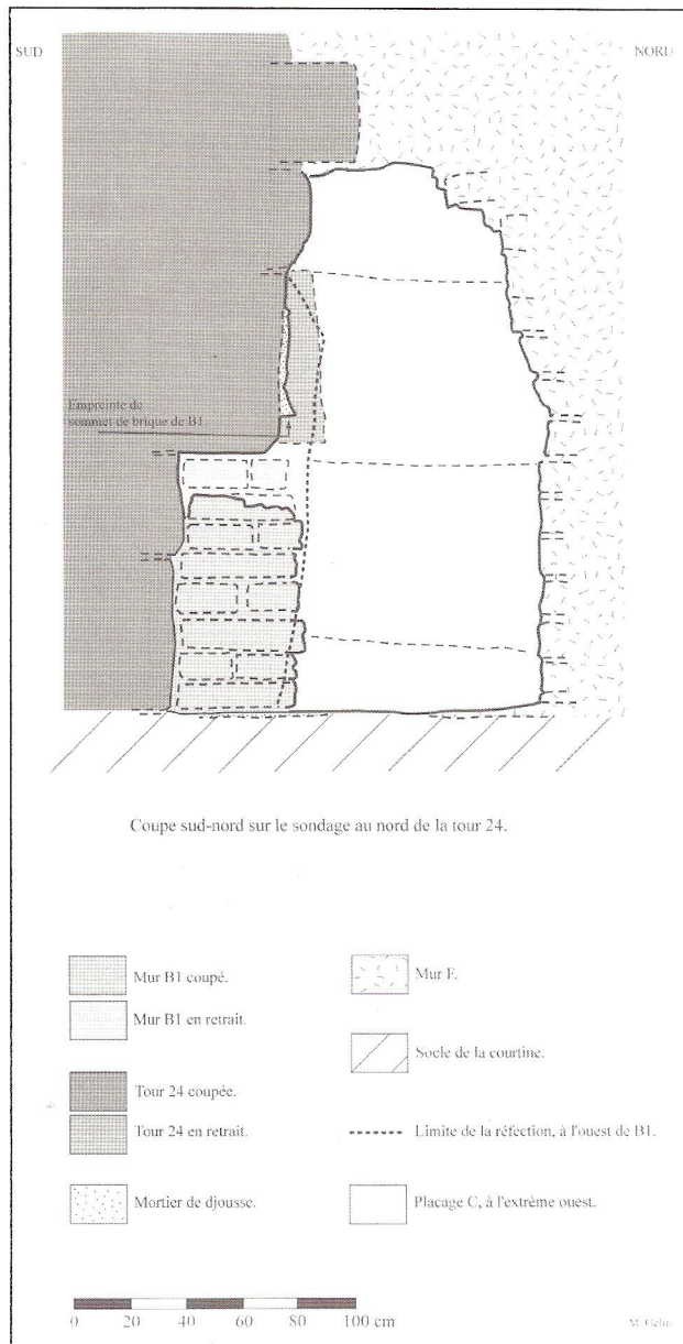
Fig. 17 – Coupe sud-nord sur les maçonneries situées dans le sondage au nord de la tour 24.
