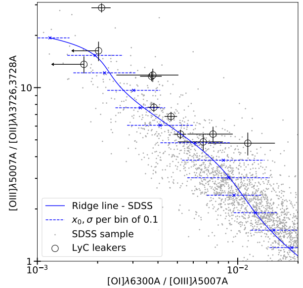
Fig. 2. O32 – O13 diagram.
