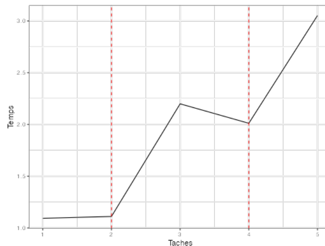
FIG. 2.2 : Temps d'exécution en parallèle de tâches nécessitant une seconde (chaque tâche est une pause d'un quart de seconde). Le nombre de tâches varie de 1 à deux fois le nombre de coeurs utilisés (égal à 2) plus une.
