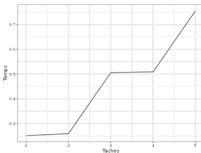
FIG. 2.2 : Temps d'exécution en parallèle de tâches nécessitant un quart de secondes (chaque tâche est une pause d'un quart de seconde). Le nombre de tâches varie de 1 à deux fois le nombre de coeurs (égal à 2) plus une.
