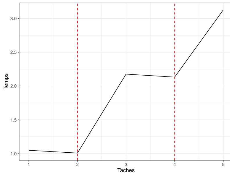
FIG. 2.2 : Temps d'exécution en parallèle de tâches nécessitant une seconde (chaque tâche est une pause d'une seconde). Le nombre de tâches varie de 1 à deux fois le nombre de cœurs utilisés (égal à 2) plus une.
