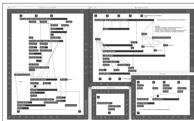
Figure 1. Une vue plongeante de quelques modules de cage.fm . Le patch est composé de plus de 500 objets (sans compter ceux compris dans des abstractions) et 30 sous-patches imbriqués sur plusieurs niveaux.
