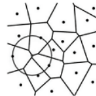
Fig. 4. Voronoi Diagram.[3]
