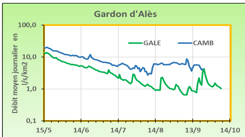
FIG.86 — DÉBITS SPÉCIFIQUES JOURNALIERS AUX STATIONS DU GALEIZON, ET DU GARDON D'ALÈS À CAMBOUS, DU 15 MAI AU 15 OCTOBRE 2019
