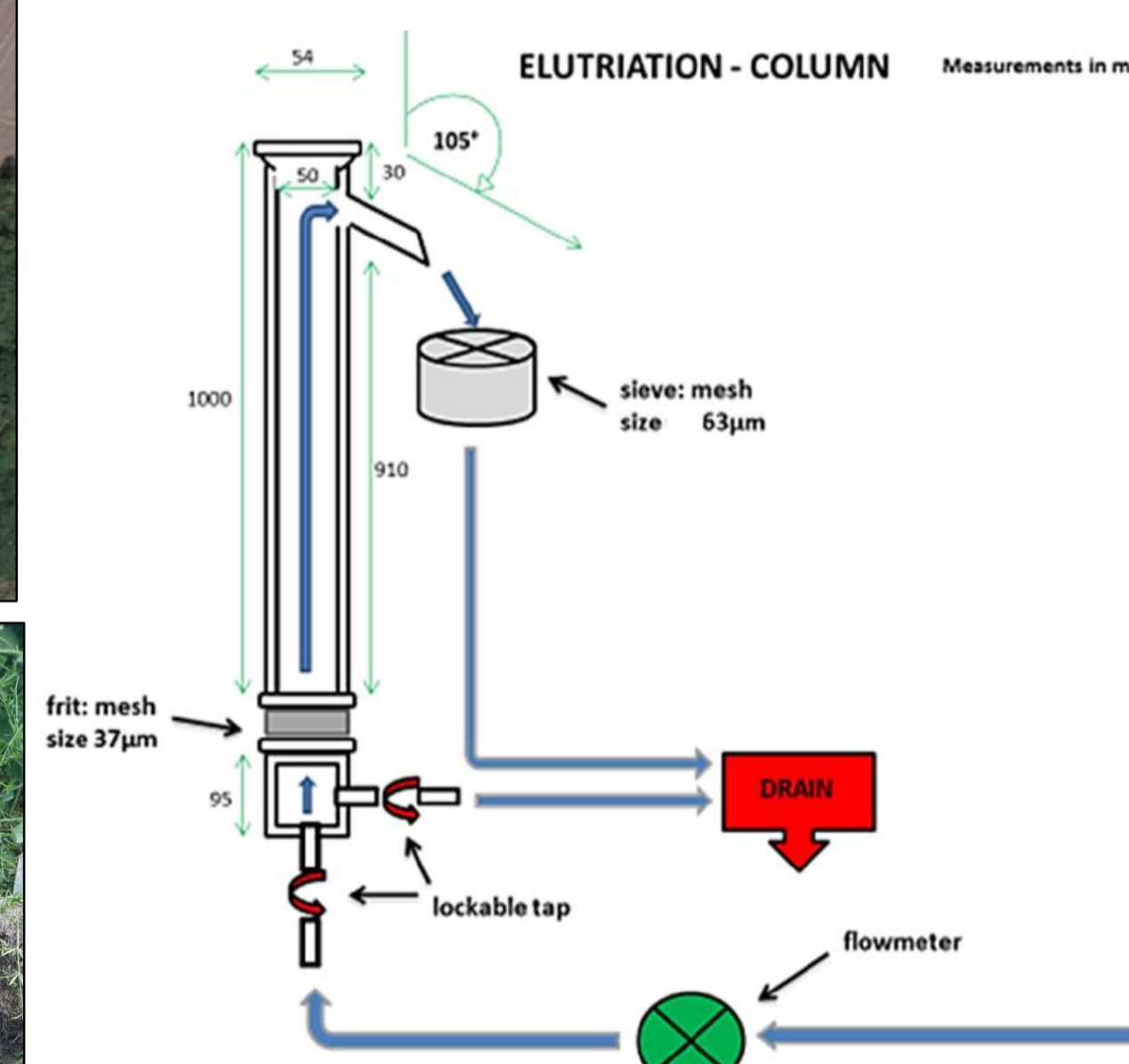
Figure 2. Schéma d'une colonne d'éluatriation (Hengstmann et al. , 2018).
