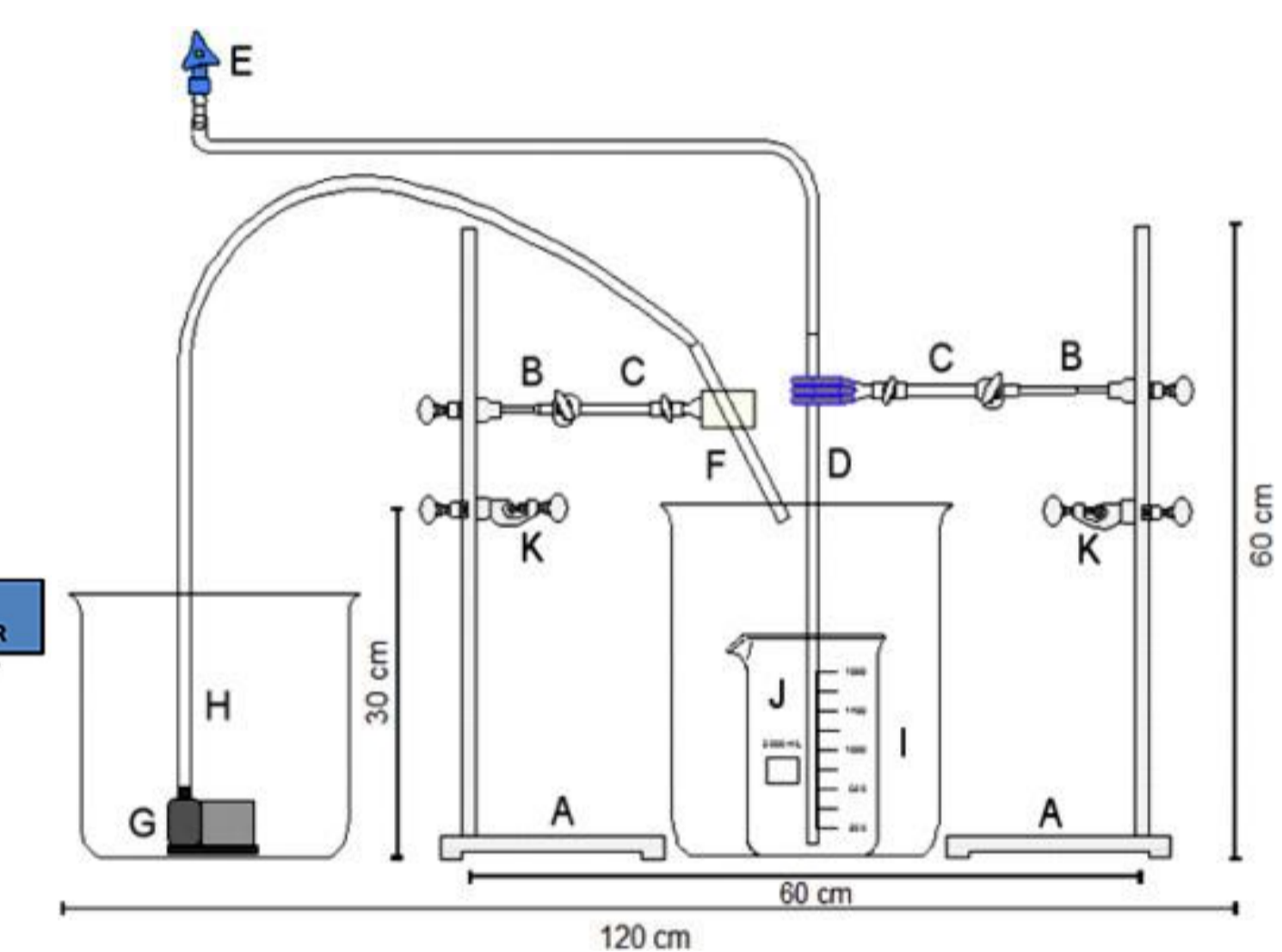
Figure 3. Schéma du dispositif « air-induced overflow » (Nuelle et al. , 2014) composé de supports (A, B, C, K) et verrerie (J, I), d'un système de bullage (D, E) et d'apport de NaCl (G, H, F).
