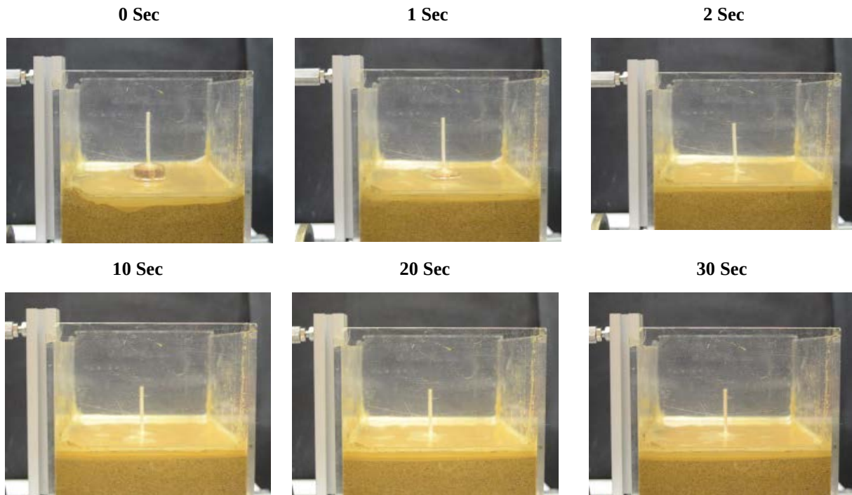
Fig.4 Capture du test effectué à 10Hz et accélération 1,56 \text{ m/s}^2 .
