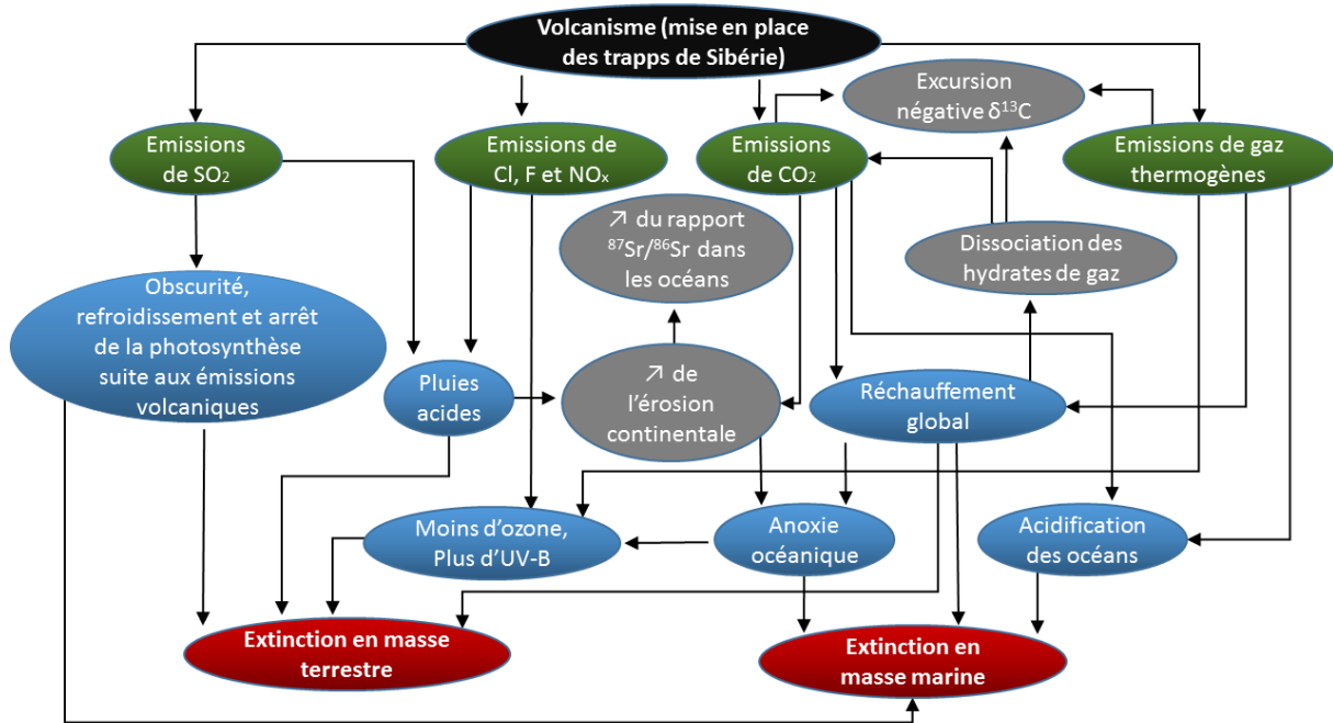
Légende Figure 1 : Diagramme résumant les relations causales à l'origine de l'extinction de masse marquant la limite Permien-Trias, il y a 252 millions d'années (modifié d'après Bond & Wignall 2014). Les cadres en bleu sont censés illustrer les "mécanismes tueurs". Si ce type de scénario complexe a le mérite de relier les causes extrinsèques entre elles, les mécanismes écologiques menant effectivement à l'extinction et l'explication de la sélectivité en sont notoirement absents.
