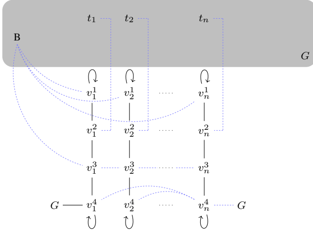
Fig. 5: Reduction of Reachability und to Coverage-init und .
