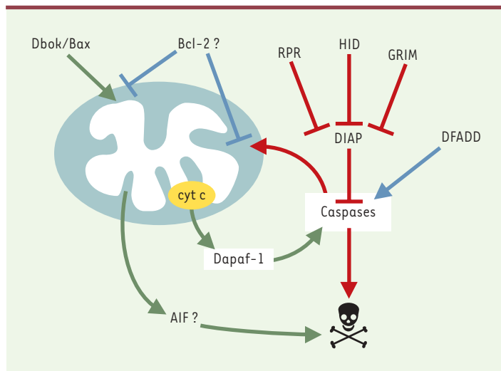
Figure 1. Modèle d'action des molécules impliquées dans le programme de mort cellulaire chez la drosophile. Les protéines RPR, HID et GRIM permettent l'activation des caspases en se liant aux protéines de type IAP ( inhibitor of apoptosis protein ), ce qui libère les pro-caspases. Bax et son homologue Dbok agiraient sur la mitochondrie, activant ainsi la voie cytochrome c/Dapaf-1 et une voie indépendante des caspases qui pourrait par exemple faire intervenir l'homologue du facteur AIF ( apoptosis inducing factor ) de mammifère. La question de l'existence d'un membre anti-apoptotique de la famille Bcl-2 chez la drosophile reste posée mais l'inhibition de l'apoptose par la protéine Bcl-2 humaine est associée au maintien de l'homéostasie mitochondriale. Enfin, la protéine DFADD, est probablement impliquée dans une voie de type récepteur de mort permettant l'activation des caspases.
