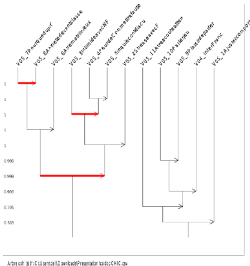
Fig. 2 Arbre cohésitif
