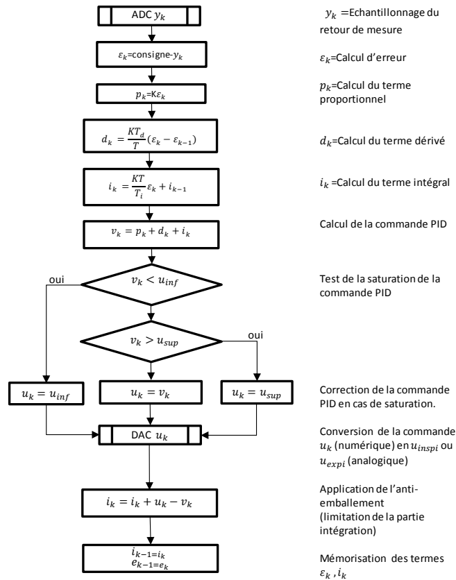
Figure 11. Algorithme de régulation PID du simulateur de respiration
