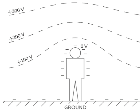
Figure 7. Distribution du potentiel électrique autour d'un humain dans un espace ouvert. Extrait de "The Feynman lectures on physics" [16]
