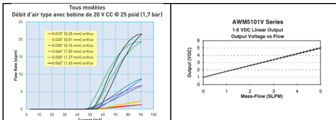
Figure 10. Caractéristiques de la vanne proportionnelle VSO (Parker) et du capteur de débit AWM5101 (Honeywell). Sources : https://www.parker.com/literature/LiteratureFiles/PrecisionFluidicsDivision/UpdatedFiles/Proportional Catalog_2013_Lowres_FR.pdf . https://sensing.honeywell.com/honeywell-sensing-airflow-awm50000-series-catalog-pages.pdf .
