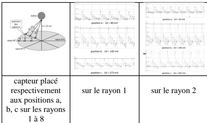
Figure 12. Réponse du capteur EPIC en fonction de la distance par rapport au fantôme
