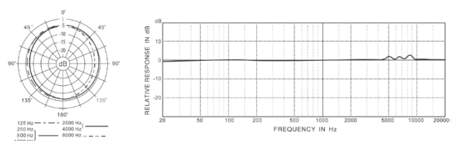
Figure 1. Réponse du microphone Behringer ECM8000
