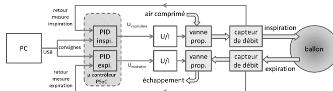
Figure 9. Synoptique du simulateur de respiration
