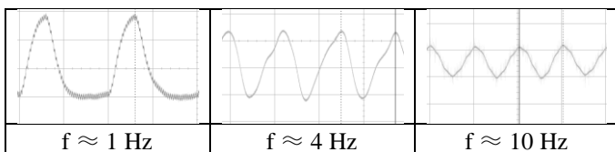
Figure 13. Réponse du capteur EPIC en fonction de la fréquence respiratoire simulée
