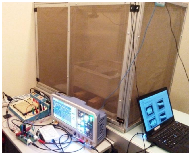
Figure 15. Cage d'hébergement dans la cage de Faraday avec l'instrumentation associée
