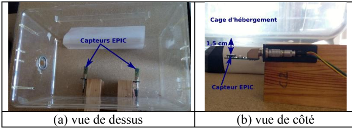
Figure 16. Positionnement des capteurs par rapport à la cage d'hébergement
