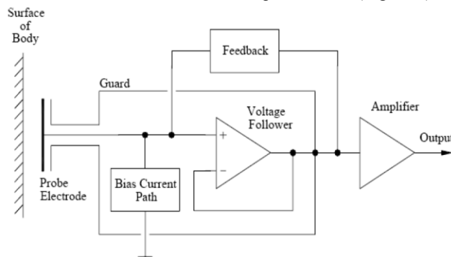
Figure 8. Schéma-bloc du capteur EPIC (Plessey Semiconductors, 2013)
