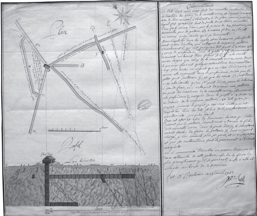
Figure 1. – Plan et profil du puits d'Arcy de la mine de Poullaouen.
