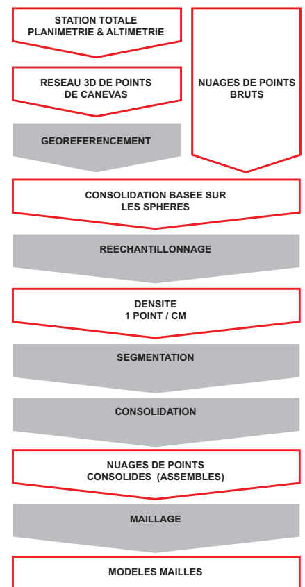
Figure 4. Chaîne de traitement des modèles 3D à partir des nuages de points bruts.
