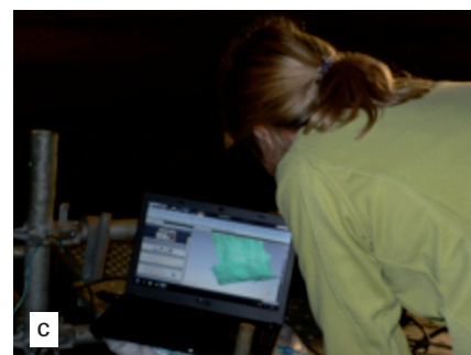
Figure 9. Numérisation d'un panneau orné du secteur 13 avec le scanner laser ScanArm de Faro ; a) Mise en place du scanner laser ScanArm ; b) numérisation du grand panneau orné du secteur 13 ; c) visualisation en temps réel des nuages de points.
