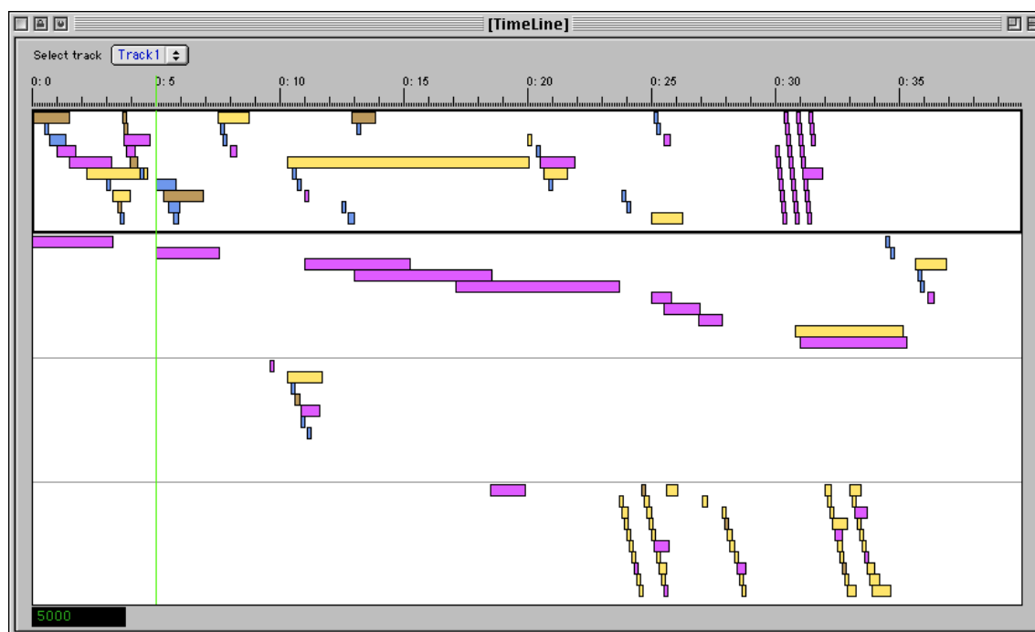
Figure 7. Visualisation selon le mode « BuffersView »
