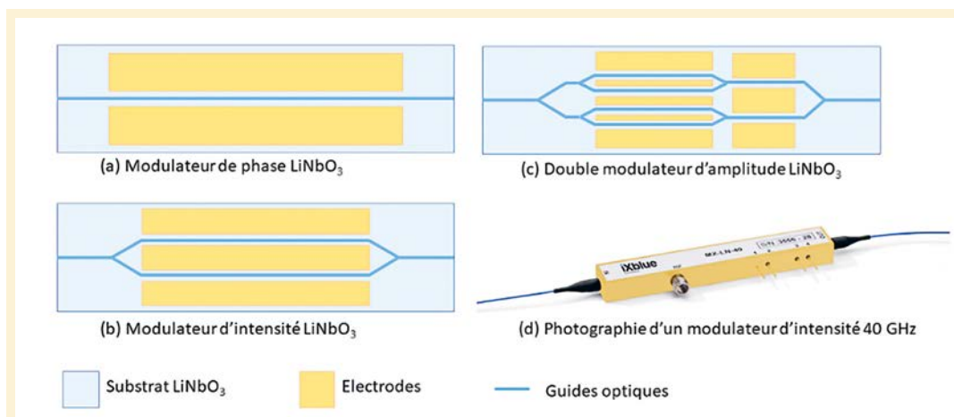
Figure 1. Différentes architectures de modulateurs intégrés \text{LiNbO}_3 . (a) Modulateur de phase. (b) Modulateur d'amplitude. (c) Double modulateur d'amplitude parallèle. (d) Photographie d'un modulateur d'amplitude commercial 40 GHz. Une description plus complète de la fabrication et des caractéristiques est donnée en références [1,2].
