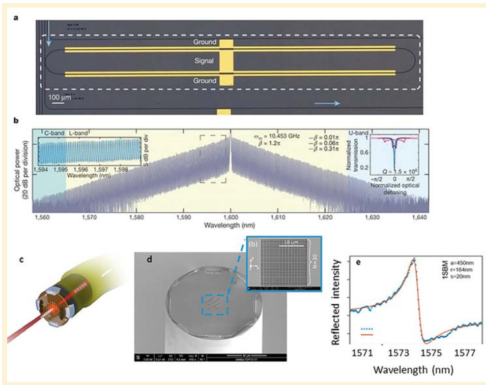
Figure 4. Composants LiNbO 3 compacts sur couches minces. (a) Deux modulateurs de phase intégrés dans un résonateur à rayon de courbure micrométrique. (b) Réponse spectrale associée à (a) : 900 peignes de fréquences répartis sur 80 nm, un record pour une tension de commande aussi faible que 10 V. (c, d, e) Cristal photonique LiNbO 3 intégré sur fibre optique : (c) schéma de principe, (d) image au microscope à balayage électrique (MEB), (e) spectre en réflexion expérimental (bleu) comparé au spectre théorique (rouge). (a), (b) Reprinted with permission from M. Zhang, Broadband electro-optic frequency comb generation in a lithium niobate microring resonator, Nature 568, 373-377 (2019), https://doi.org/10.1038/s41586-019-1008-7 . (c), (d), (e) Adapted by permission from V. Calero, An ultra wideband-high spatial resolution-compact electric field sensor based on Lab-on-Fiber technology, Scientific reports , 9: 8058, https://doi.org/10.1038/s41598-019-44644-y
