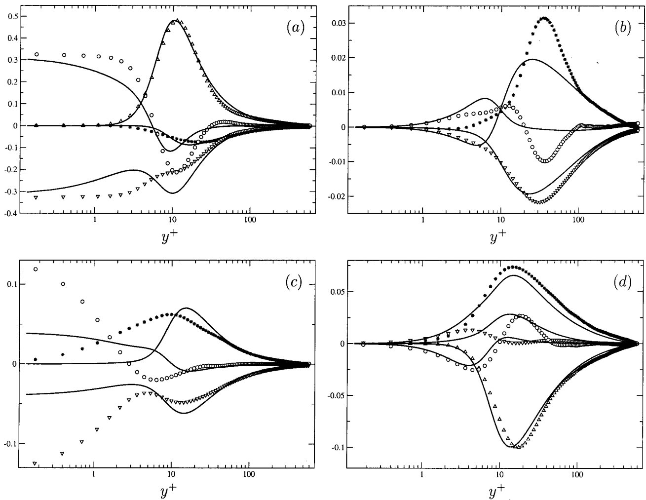
FIG. 5. Channel flow at Re_\tau=590 . Budgets of the Reynolds stresses. (a) \overline{u'u'} ; (b) \overline{v'v'} ; (c) \overline{w'w'} ; (d) \overline{uv'} . Symbols: DNS ( \Delta Production P_{ij} ; * Redistribution \phi_{ij}^* ; \nabla Dissipation -\varepsilon_{ij} ; \circ Total diffusion D_{ij}^v + D_{ij}^T ). — Elliptic blending model.
