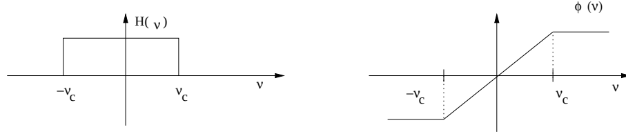
Figure V.1: Réponse d'un filtre idéal passe-bas de phase linéaire de fréquence \nu_c
