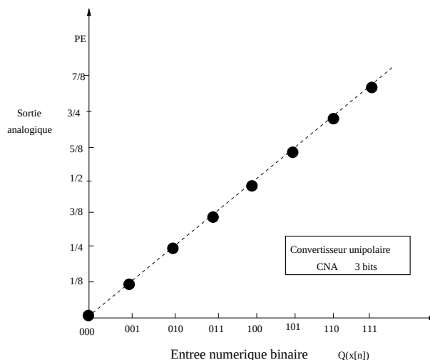
Figure I.25: Caractéristique de transfert d'un CNA sur 3 bits.
