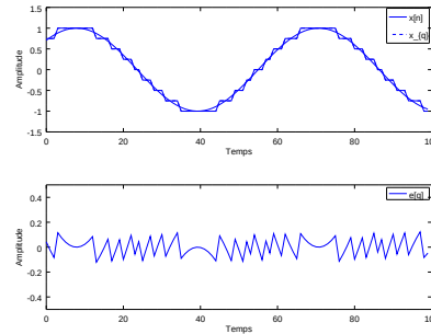
Figure I.19: Quantification d'un signal sinusoïdal sur 5 bits par la méthode de l'arrondi. L'erreur de quantification du signal est extraite juste après.
