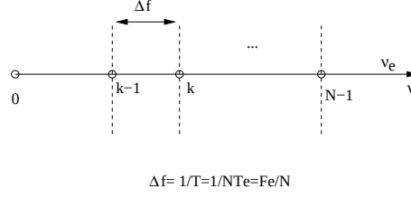
Figure II.1: Résolution \Delta\nu des échantillons spectraux. Chaque échantillon spectral k de DFT est espacé de \Delta f = \frac{\nu_e}{N} de [0; \nu_e] .
