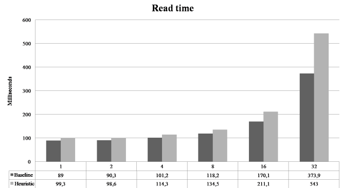
Figura 6. Média do tempo gasto na leitura e alocação de memória
