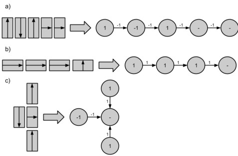
Figura 3. Representação do circuito no grafo.
