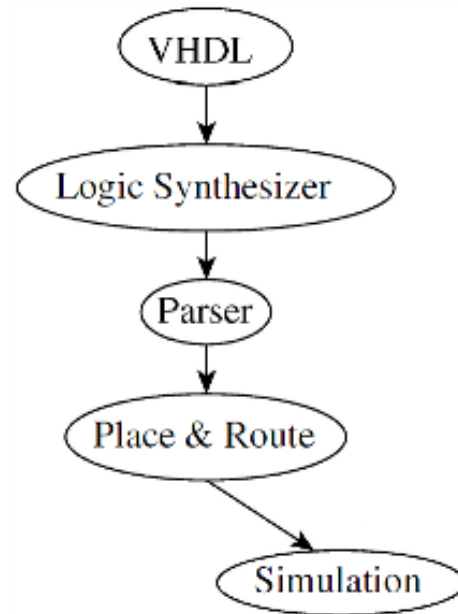
Figura 2. Fluxo de projeto da ferramenta ToPoliNano
