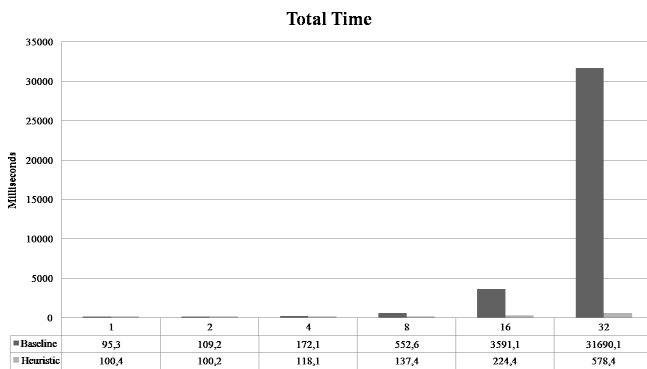
Figura 5. Média do tempo gasto em 10 execuções para cada somador.
