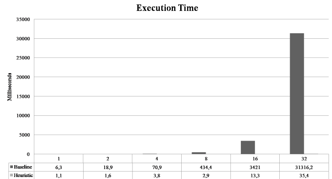
Figura 7. Média do tempo gasto para calcular o valor de todos os ímãs.
