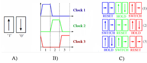
Figura 1. A) Representação de um ímã e seu vetor de magnetização. B) Sinais de clock. C) Ímãs em três zonas e seus estados.
