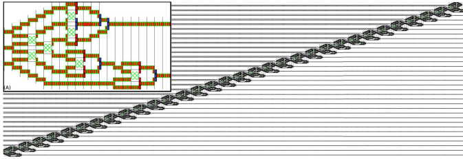
Figura 4. Em foco um somador de 1 bit. Na imagem maior o somador de 32 bits.
