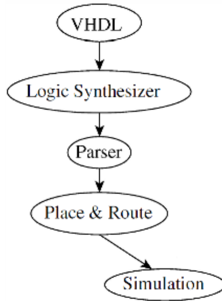
Figura 2. Fluxo de projeto da ferramenta ToPoliNano
