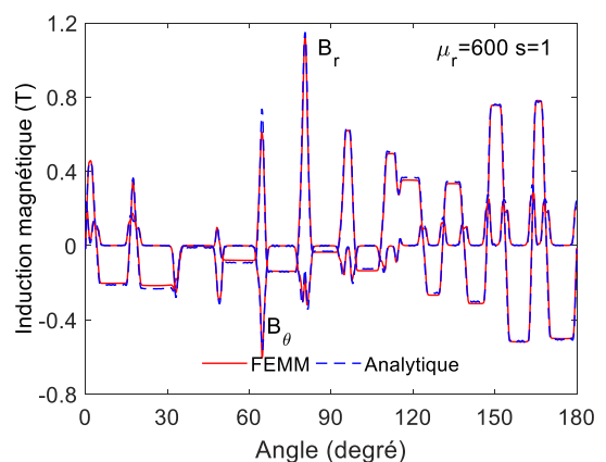
Fig. 5. Composante r et \theta de l'induction magnétique au milieu de l'entrefer pour \mu_r = 600 et s = 1 .
