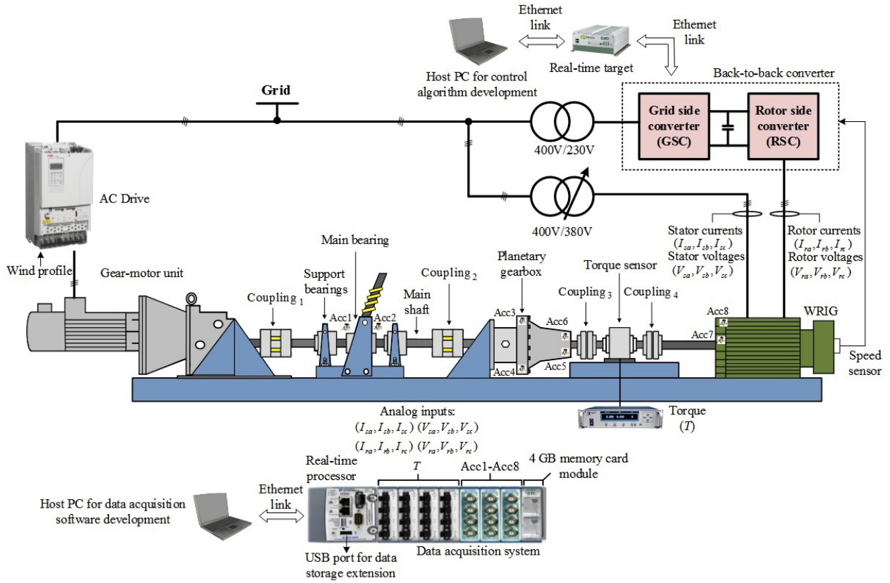
Fig. 3. Banc d'essai à échelle réduite simulant le fonctionnement d'une éolienne.
