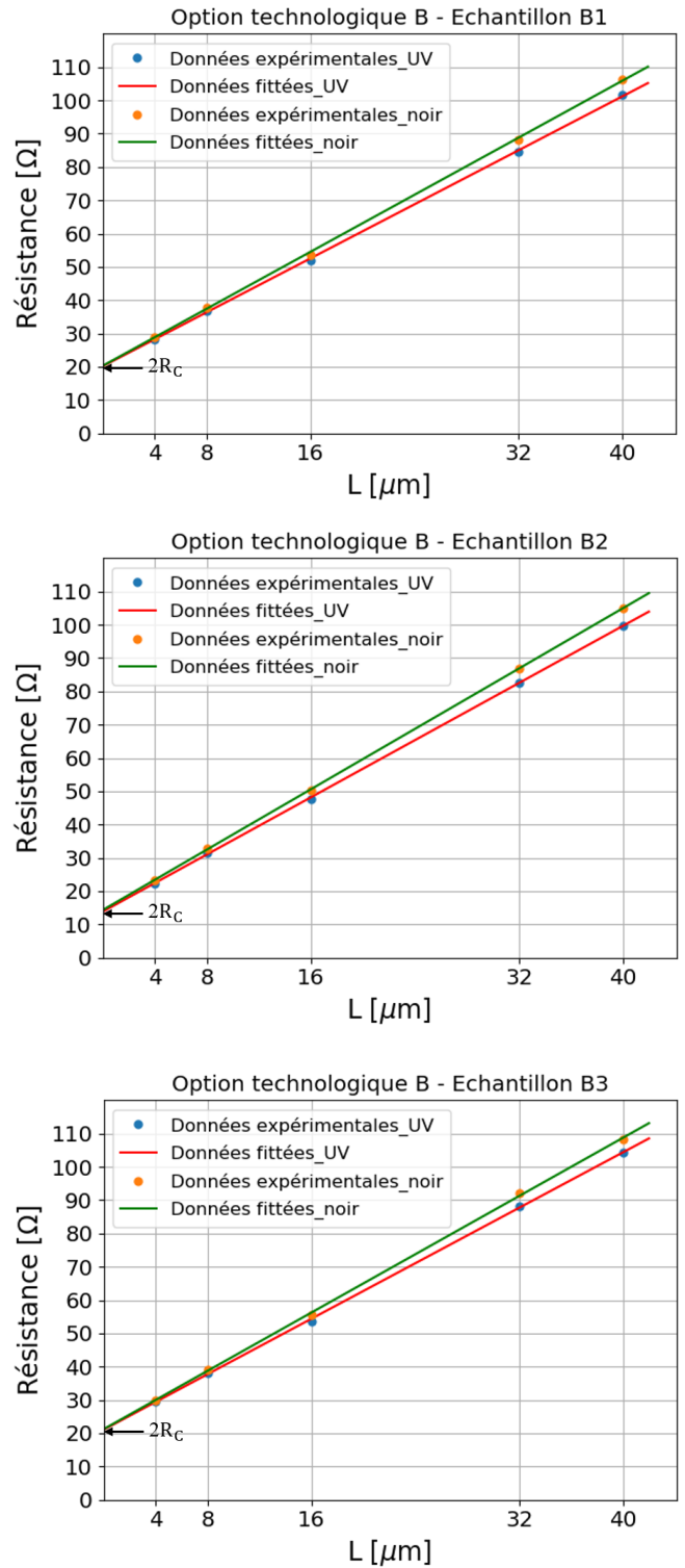
Fig. 6. Caractéristiques R(L) extraites, pour 3 échantillons, avec l'option technologique B.
