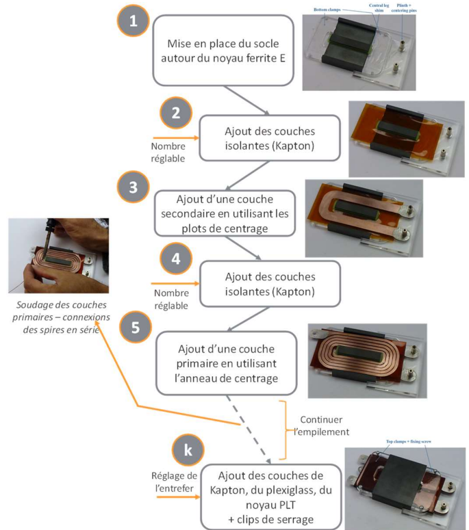
Fig. 6. Processus d'assemblage.
