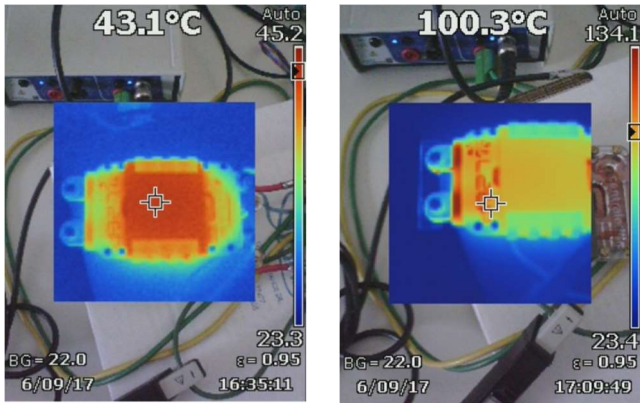
Fig. 10. Mesure de la température : (a) Essais à vide et (b) Essai avec court-circuit au secondaire.
