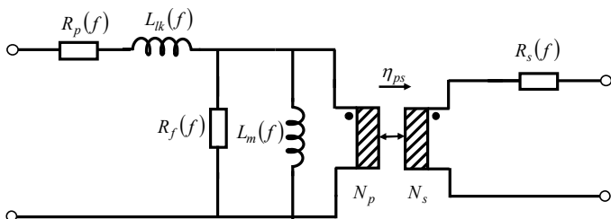
Fig. 9. Schéma équivalent du transformateur à 2 enroulements (parties magnétique et pertes).
