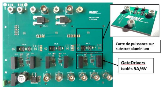
Figure 13 : Onduleur GaN 2kW triphasé 2 niveaux
