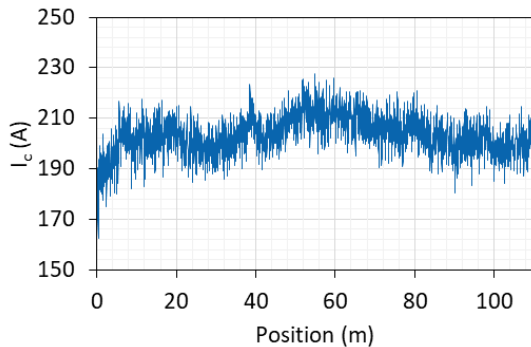
Fig. 2: Répartition des valeurs de courant critique le long d'un ruban SHTC de 4 mm obtenues par mesure inductive à 77 K en champ propre (données SuperOx®)
