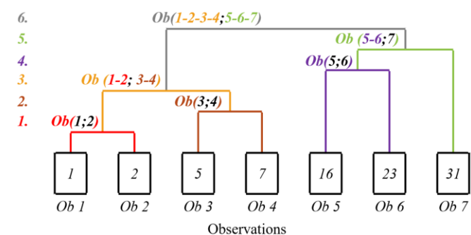
Fig. 2. Illustration de l'algorithme de CAH
