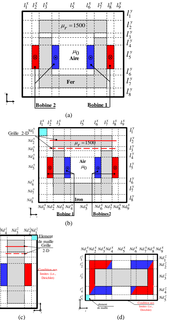
Fig. 7. Dispositif électromagnétique statique à noyau en U dans les différents plans.
