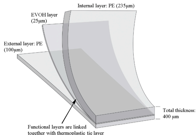
Fig. 1. Example of PE bag.
