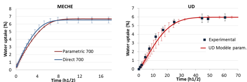
Fig.3 Comparaison de la prise en eau obtenue pour les modèles réaliste et paramétrique à l'échelle de la mèche / Comparaison entre expérience et modèle à l'échelle « UD ».
