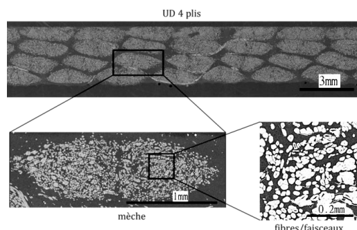
Fig. 1 : Organisation multi-échelles du composite UD lin/polyester.
