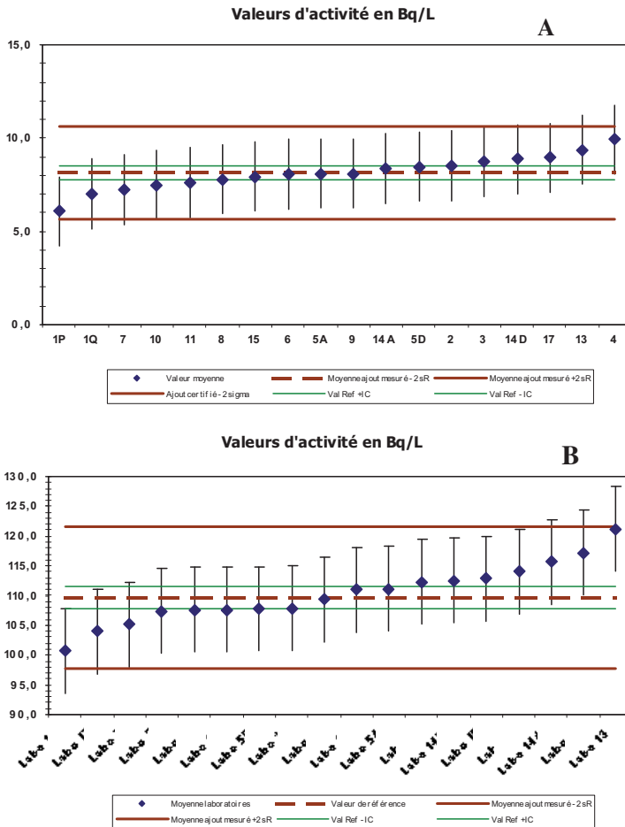
Figure 5 – Résultats d'une intercomparaison (18 participants) d'analyse d'eau tritiée avec 2 concentrations. (A) 8 Bq.L -1 , (B) 110 Bq.L -1 .
