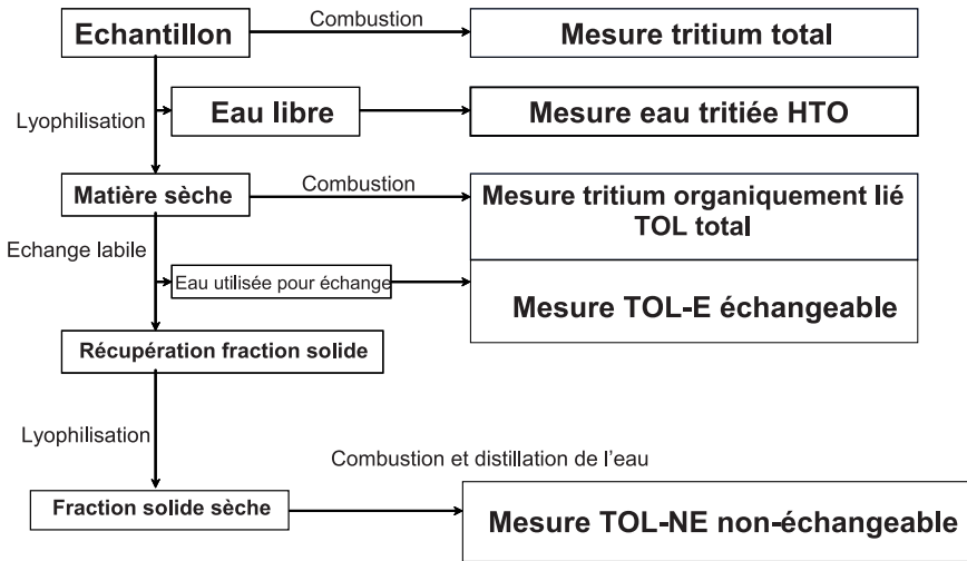
Figure 1 – Schéma d'analyse du tritium dans les échantillons de l'environnement. Tritium analysis diagram in environmental samples.
