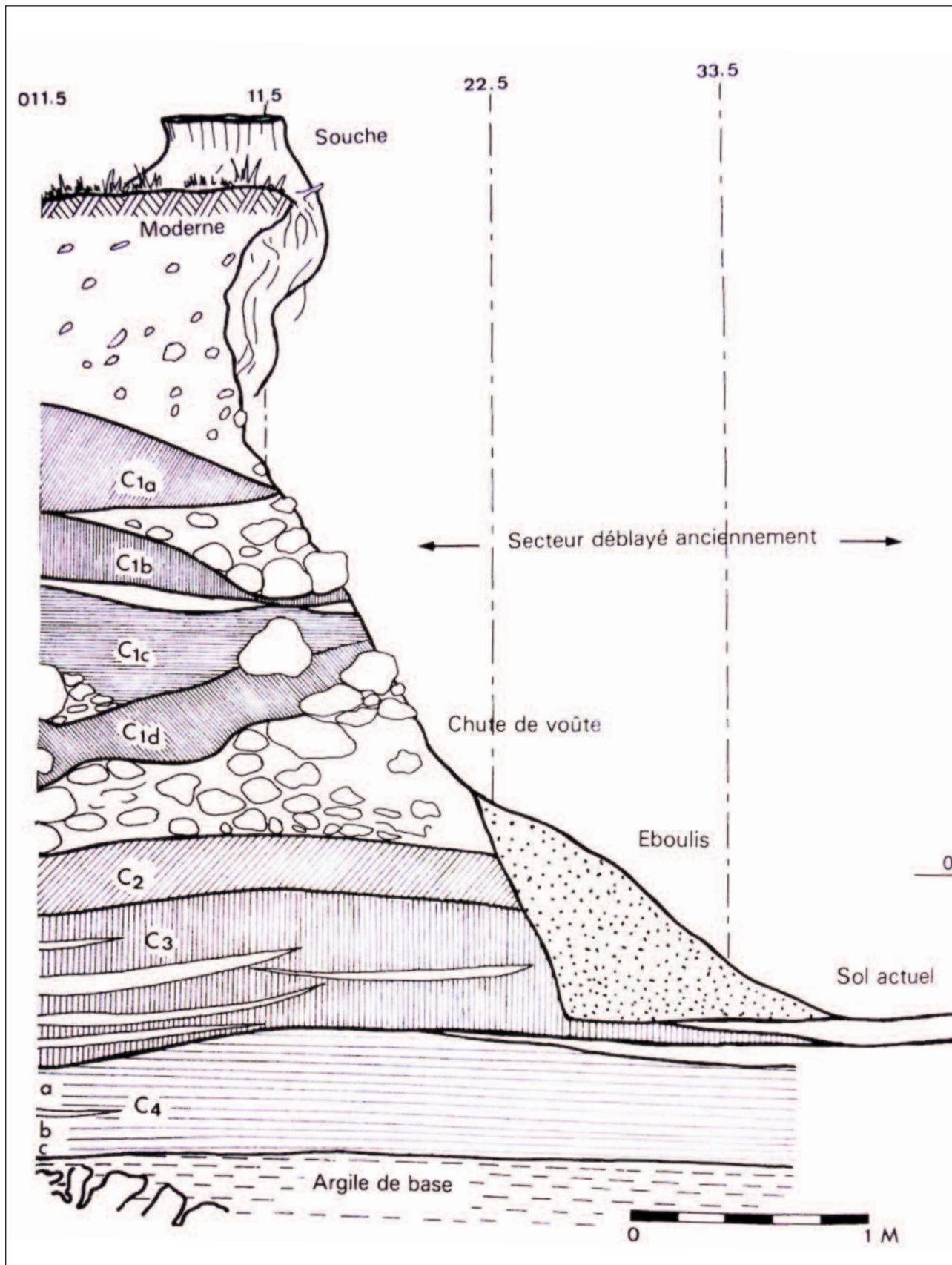
Figure 4 - Stratigraphie du gisement du porche d'entrée de la grotte de Rouffignac. Coupe frontale. (© Relevés et dessin de C. Barrière).
