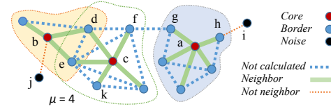
Fig. 1. Basic idea of anySCAN
