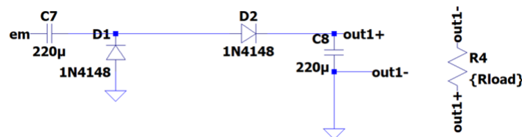
(d) Standard silicon diodes interface
