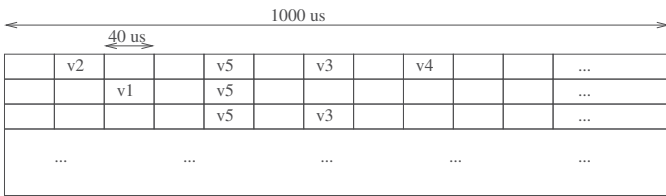
Fig. 5. Table with one slot per BAG per VL
