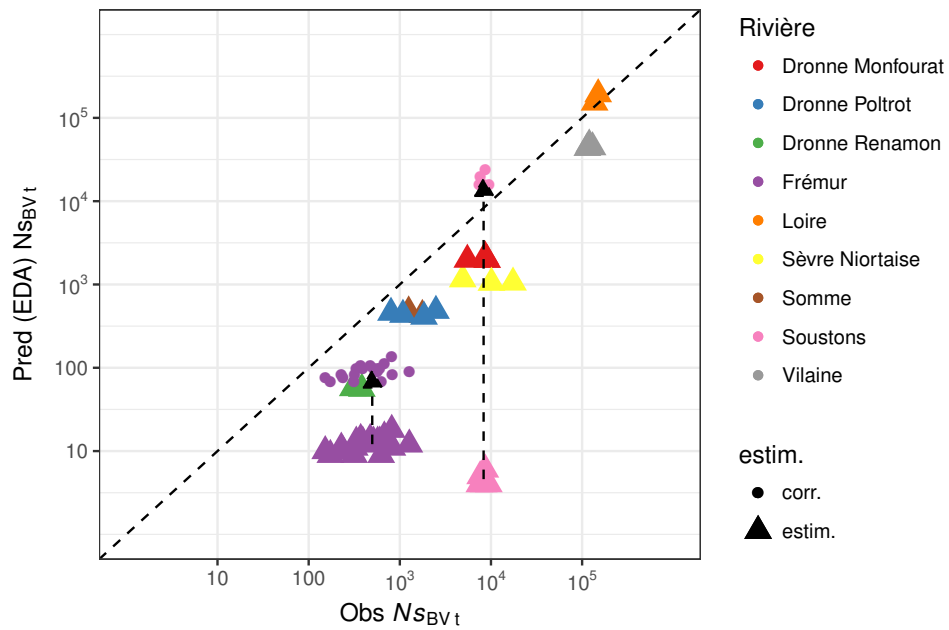
FIGURE 4 – Comparaison des productions estimées par EDA ( \widehat{N}_{s_{BV,t_a}} ) et des productions des bassins versants des rivières index et des pêcheries d'argentées N_{s_{BV,t}} . Deux cas sont considérés, ( \blacktriangle ) estimation de la production totale annuelle, dans le cas du Frémur et de Soustons, les estimations d'EDA ( \bullet ) sont augmentées pour prendre en compte les surfaces en eau des lacs et des étangs, très importantes sur ces bassins et qui ne sont pas estimées dans le RHT.
