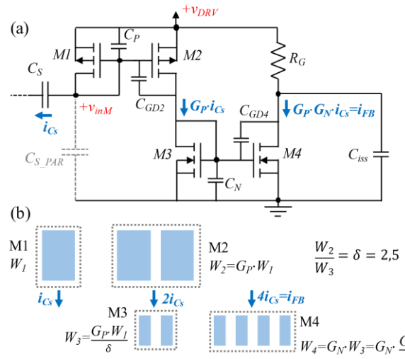
Fig. 4. (a) Miroirs de courant avec deux étages d'amplification de courant représentés avec leurs capacités intrinsèques. (b) Layout considérant un facteur de forme de 2.5 entre les transistors NMOS et PMOS ( G_P=2 et G_N=2 ).
