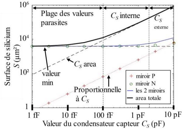
Fig. 10. Surface silicium de la boucle de rétroaction fonction de C_S pour une atténuation donnée (produit G \cdot C_S = 10 pF constant).
