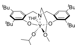
Y-O i Pr
