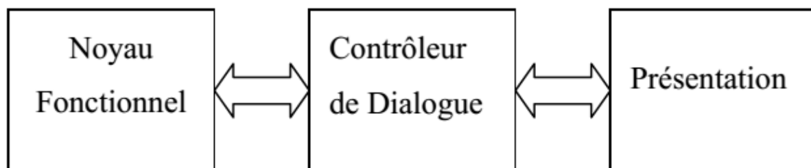
Fig.3.8 Le modèle de Seeheim [4].
