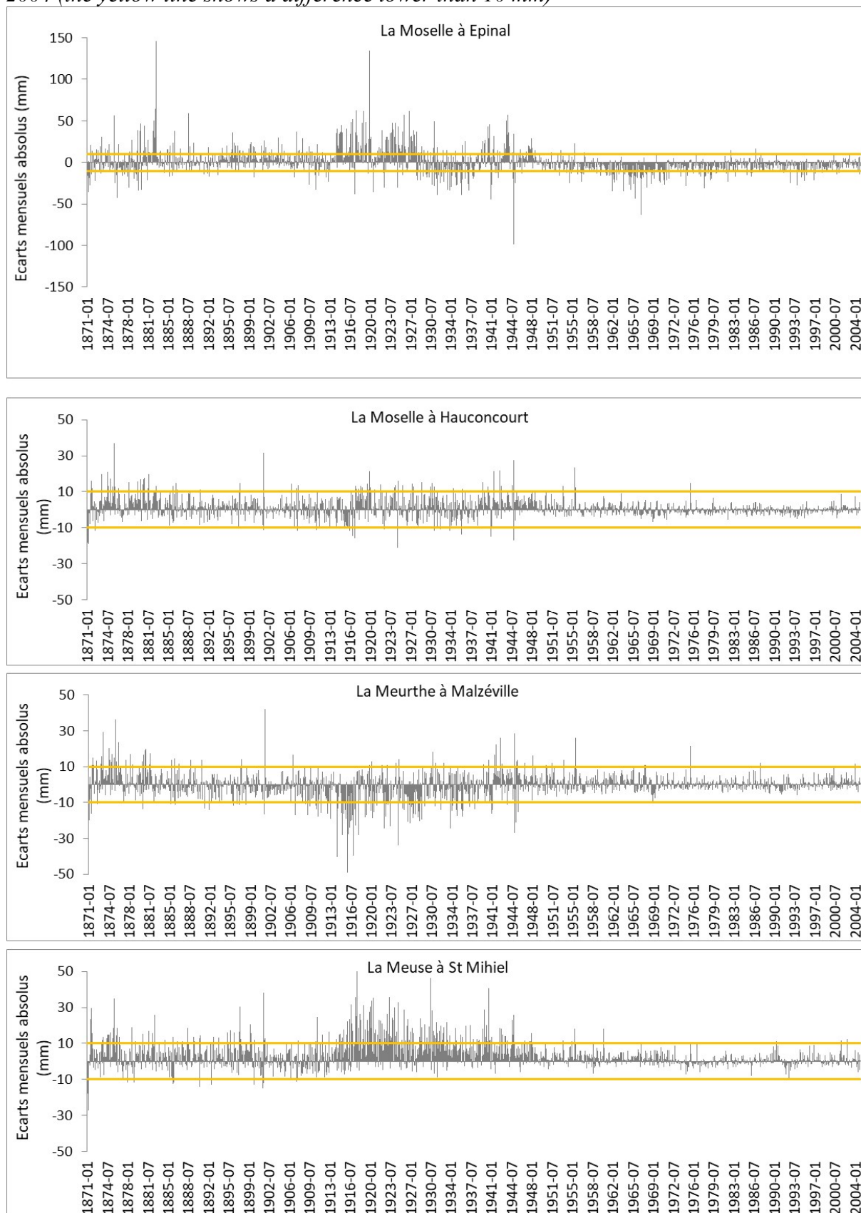
Figure 10 : Écarts mensuels absolus (en mm) entre RECRET et FYRE Daily calculés sur la période 1871-2004 (le rail jaune correspond à un écart absolu inférieur à 10 mm)
