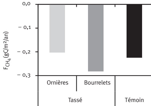
FIGURE 2 MOYENNE SUR DEUX ANNÉES DU FLUX NET ANNUEL DE MÉTHANE À L'INTERFACE SOL-ATMOSPHÈRE EN FORÊT DES HAUT-BOIS (Azerailles, Meurthe-et-Moselle), SUR LE TRAITEMENT TÉMOIN (non tassé, en noir) ET DANS LES ORNIÈRES (gris clair) OU LES BOURRELETS (gris moyen) DU TRAITEMENT TASSÉ
